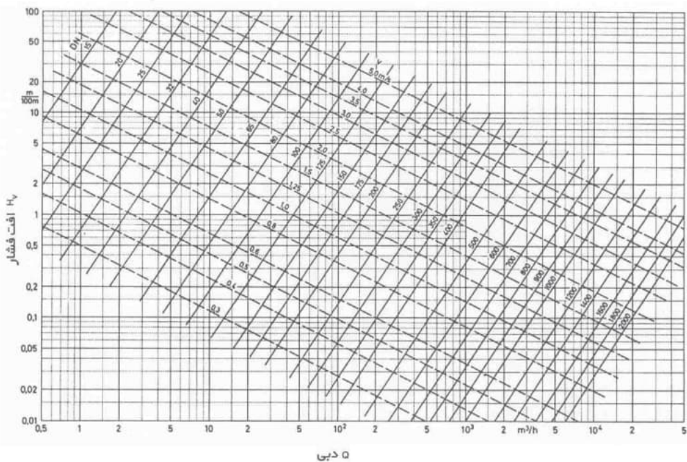
شکل ۱۲- افت فشار در لوله‌های مستقیم (چدن خاکستری کار نکرده) از قطر ۱۵ میلی‌متر تا ۲۰۰۰ میلی‌متر و دبی ۰.۵ تا ۵۰۰۰۰ مترمکعب در ساعت.
