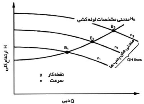
شکل ۱۸- تأثیر تغییر سرعت دورانی
