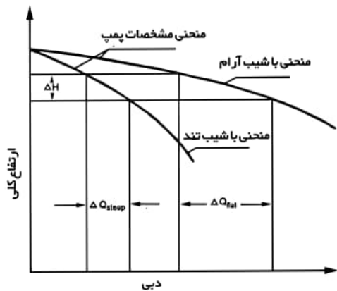
شکل ۴- منحنی مشخصات با شیب تند و آرام.
