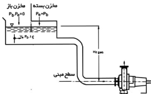
شکل ۱۱ - NPSH_{AV} موجود در شرایطی که پمپ پایین‌تر از سطح مایع قرار دارد.
