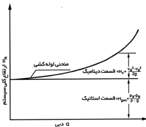
شکل ۵- منحنی مشخصات لوله کشی (سیستم).
