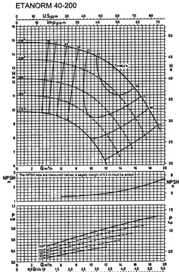
شکل ۳- منحنی مشخصات پمپ سانتریفیوژ.
