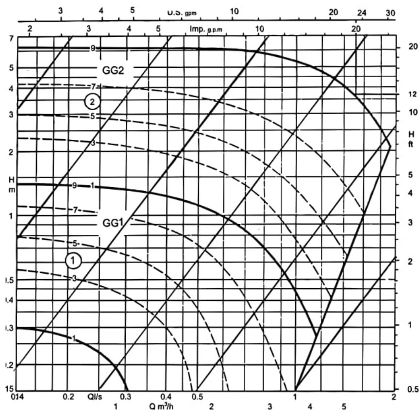
شکل ۳۴- منحنی مشخصات پمپ‌های GG1 و GG2.
