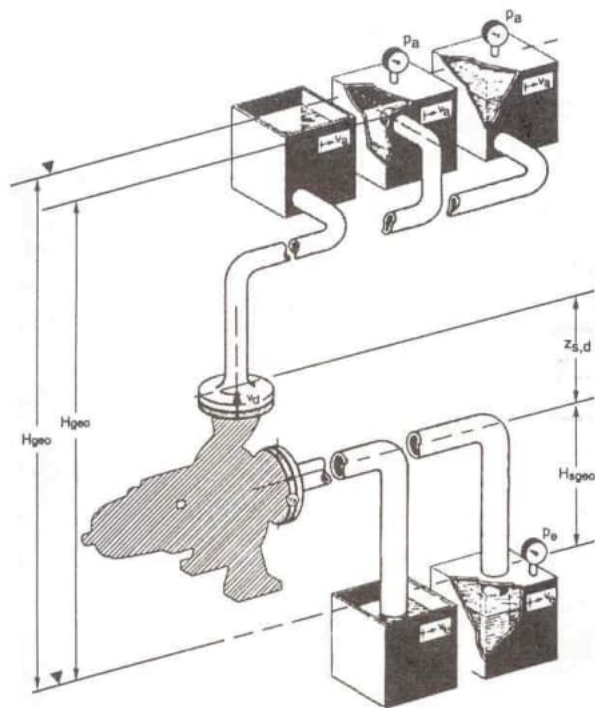
شکل ۱- مکش (پمپ بالاتر از سطح مایع در طرف مکش قرار دارد).
