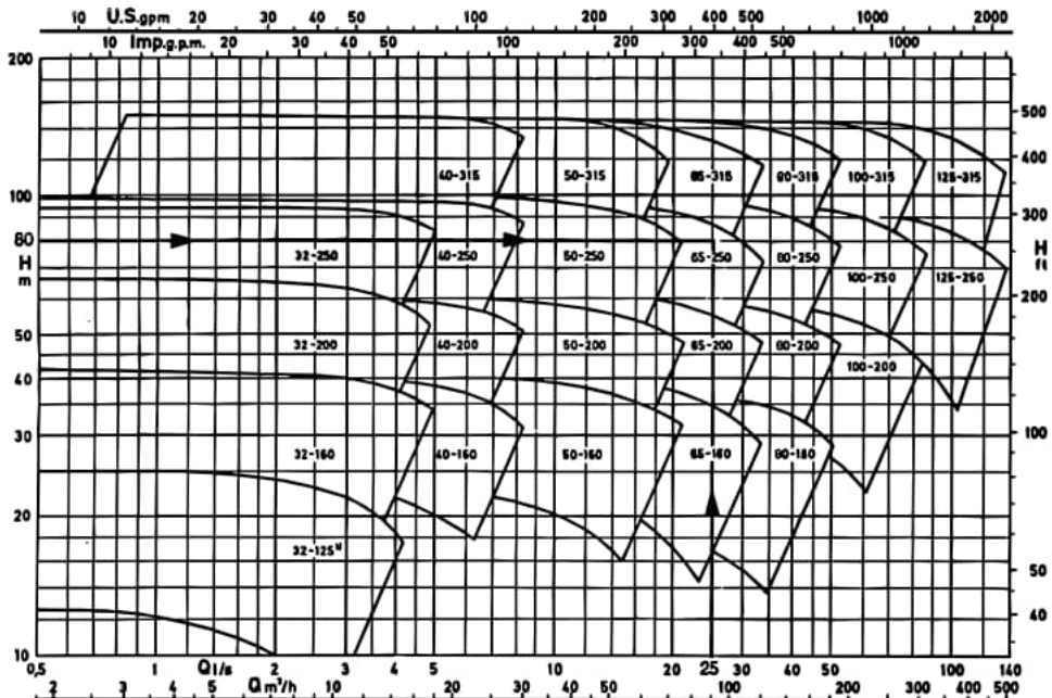
شکل ۲۴- پمپ های شیمیایی CPK (جدول کلی انتخاب) دور n = 2900 \text{ 1/min}
