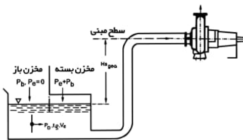
شکل ۱۰ - NPSH_{AV} موجود در شرایطی که پمپ بالاتر از سطح مایع قرار دارد.
