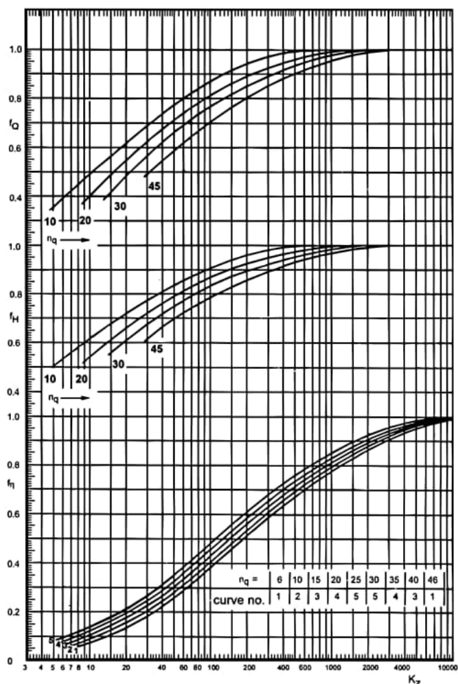
شکل ۲۱-جدول تعیین ضرایب تبدیل f_H ، f_Q و f_{\eta} برای پمپاژ مایعات با ویسکوزیته زیاد.
