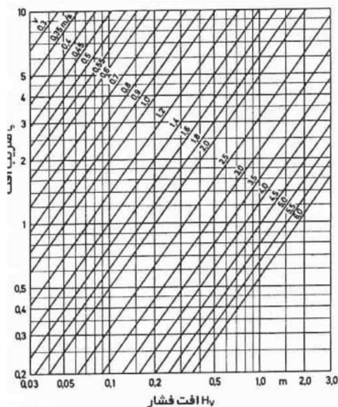
شکل ۱۳- ضرایب افت فشار برای اتصالات مختلف. شکل ۱۴- محاسبه افت فشار در شیرها و اتصالات.
