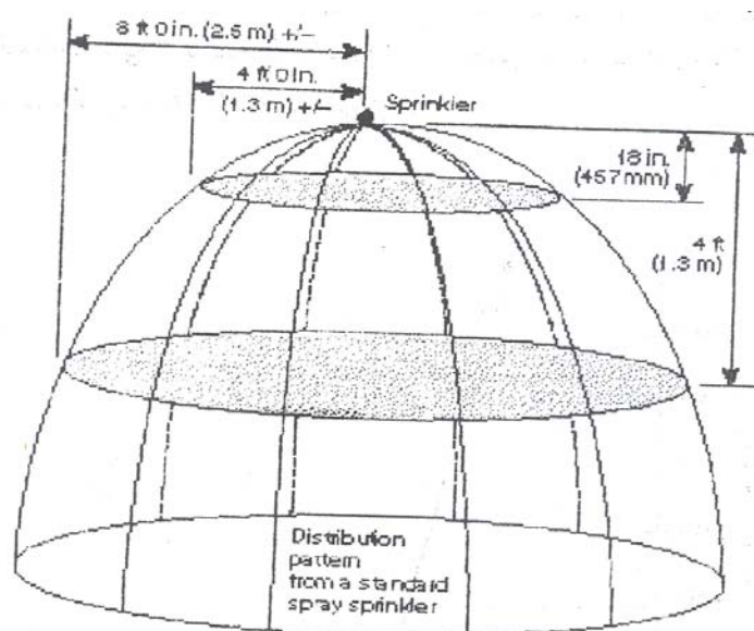
شکل ۴-۱ شعاع پوشش افشانه ها بر حسب ارتفاع
