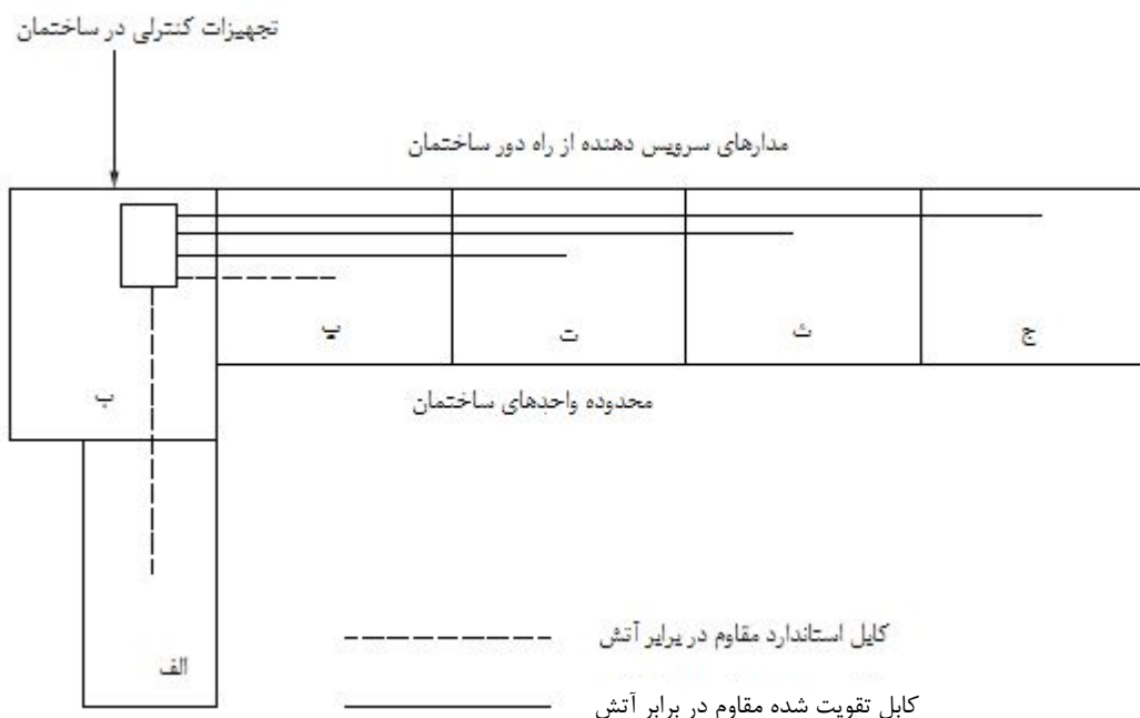
شکل ۱۴- مثالی از سیستم اعلام حریق شبکه شده
