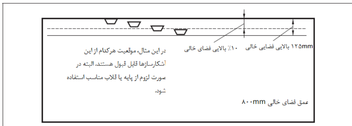
شکل ۷ - آشکارسازهای در ۱۰٪ بالایی یک فضای خالی
