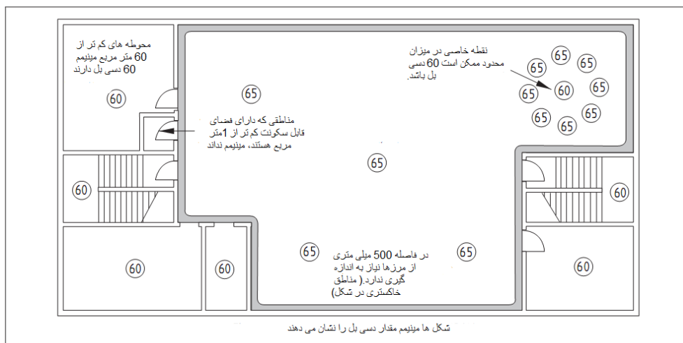
شکل ۴ - تراز فشارصوت
