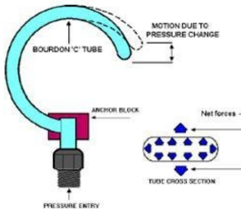
شکل ۳-۲ روش اندازه گیری بوردن تیوب از نوع C
