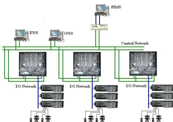
شکل ۵-۹ ساختار کنترلی غیرمتمرکز (Distributed Control System)
