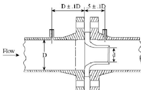
شکل ۳-۵ نازل
