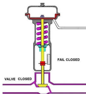
شکل ۷-۳ شیر کنترل نرمال - بسته ۱ ، وقتی باز بسته است که فشار دیافراگم به فشار اتمسفر کاهش یابد.
