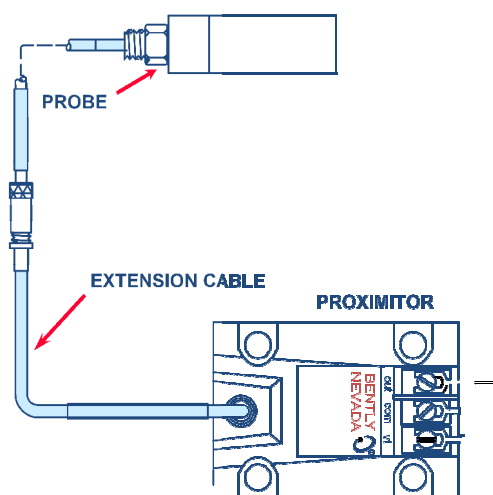
شکل ۴-۱۷ اجزاء اصلی ترانسدیوسر پراکسی میتری
