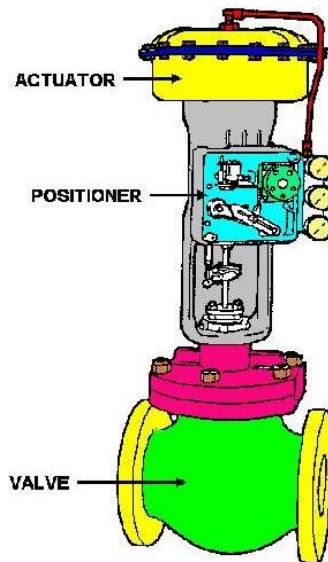
شکل ۷-۱۹- شیر کنترل و پوزیشنر
