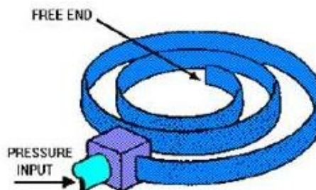
شکل ۴-۲ روش اندازه گیری بوردن تیوب از نوع مارپیچی یا حلزونی
