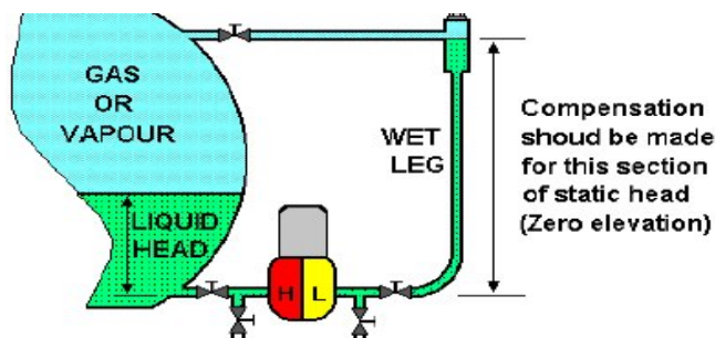
شکل ۴-۸ ارتفاع سنج اختلاف فشاری برای حالت مخزن سرپسته
