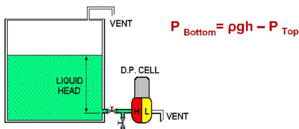
شکل ۴-۵ D.P.cell متصل شده به یک مخزن روباز
