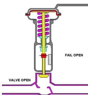
شکل ۷-۲ شیر کنترل نرمال - باز ۴ ، وقتی باز است که فشار دیافراگم به فشار اتمسفر کاهش یابد.
