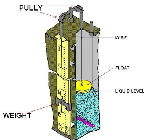
شکل ۴-۲ ارتفاع سنج شناوری
