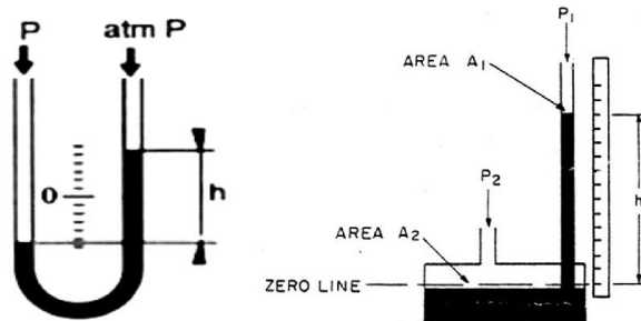
شکل ۲-۲ روش اندازه گیری مانومتر
