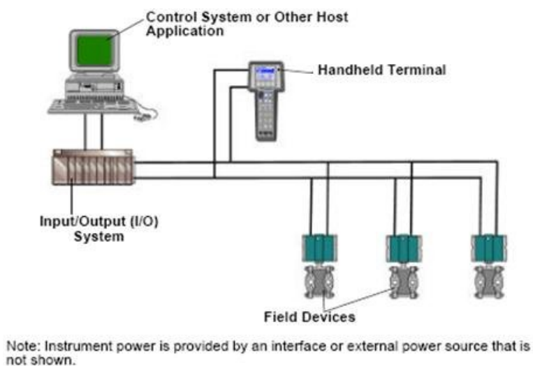
شکل ۶-۸ شبکه HART بصورت Multidrop
