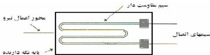
شکل ۹-۲ شمای کلی استرین گیج
