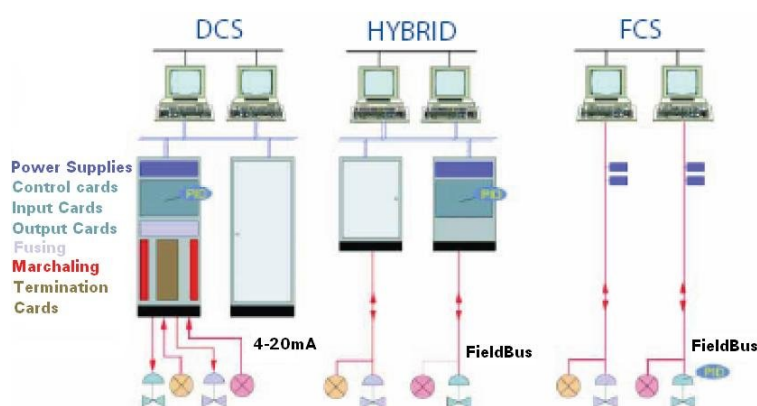
شکل ۵-۱ مقایسه ی ساختاری سیستم های کنترل DCS، FCS و Hybrid
