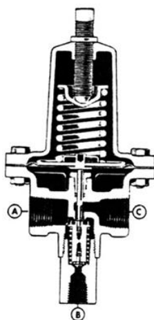
شکل ۷-۲۴ شیر حبسی که برای نگهداری شیر در آخرین موقعیت آن هنگام بروز خطا در هوای تغذیه استفاده می شود.
