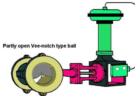
شکل ۷-۹- شیر توپی و ساختار اکچویتور دیافراگمی
