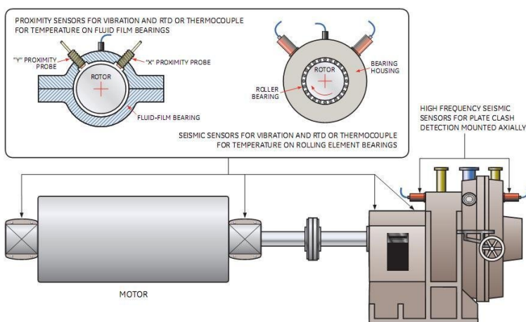
شکل ۴-۱۶ تجهیز دوار و پروپ های مربوطه
