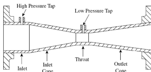
شکل ۴-۵ لوله ی ونچوری
