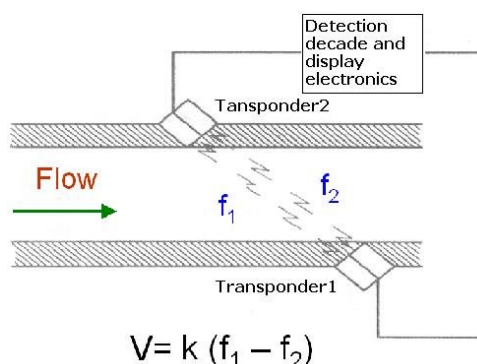
شکل ۹-۵ فلومتر اولتراسونیک
