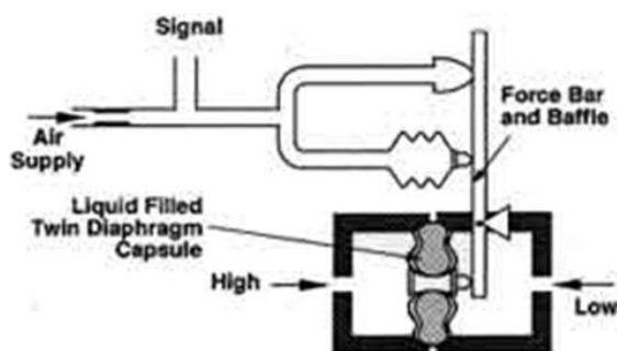
شکل ۶-۱ ترانسمیتر اختلاف فشار نیوماتیکی
