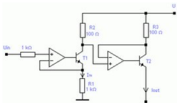
شکل ۶-۲ مبدل ولتاژ به جریان
