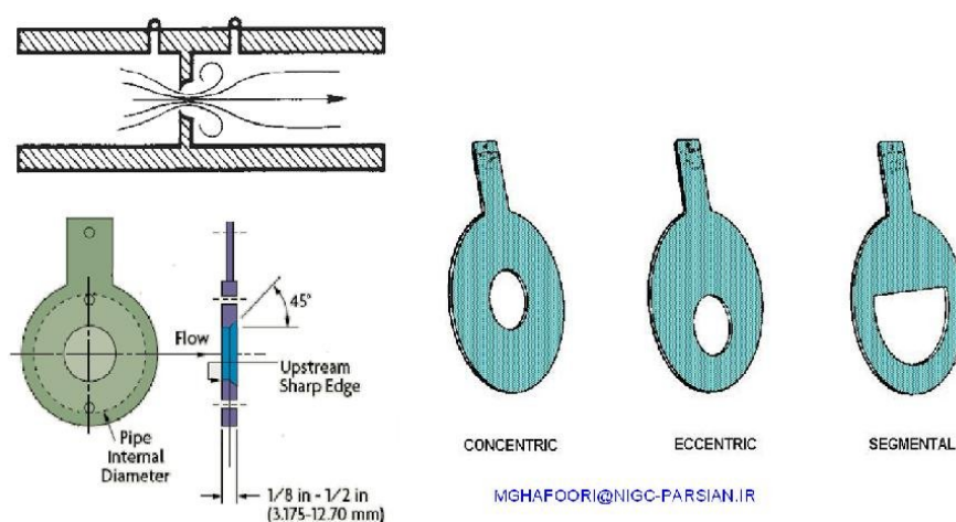
شکل ۵-۱ اشکال مختلف اریفیس
