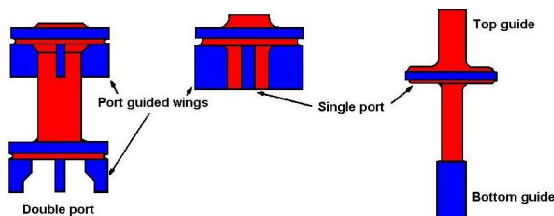
شکل ۷-۱۱- پلاگ‌های مشخصه بازکردن سریع
