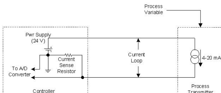
شکل ۳-۶ شماتیک ترانسمیتر ۴-۲۰ mA
