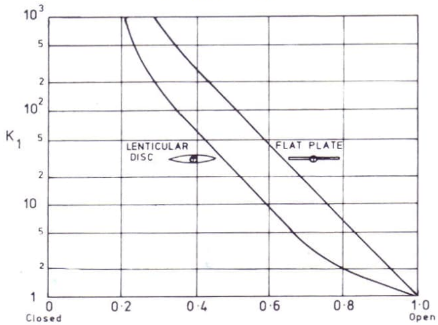
نمودار ۳ شیر پروانه ای
