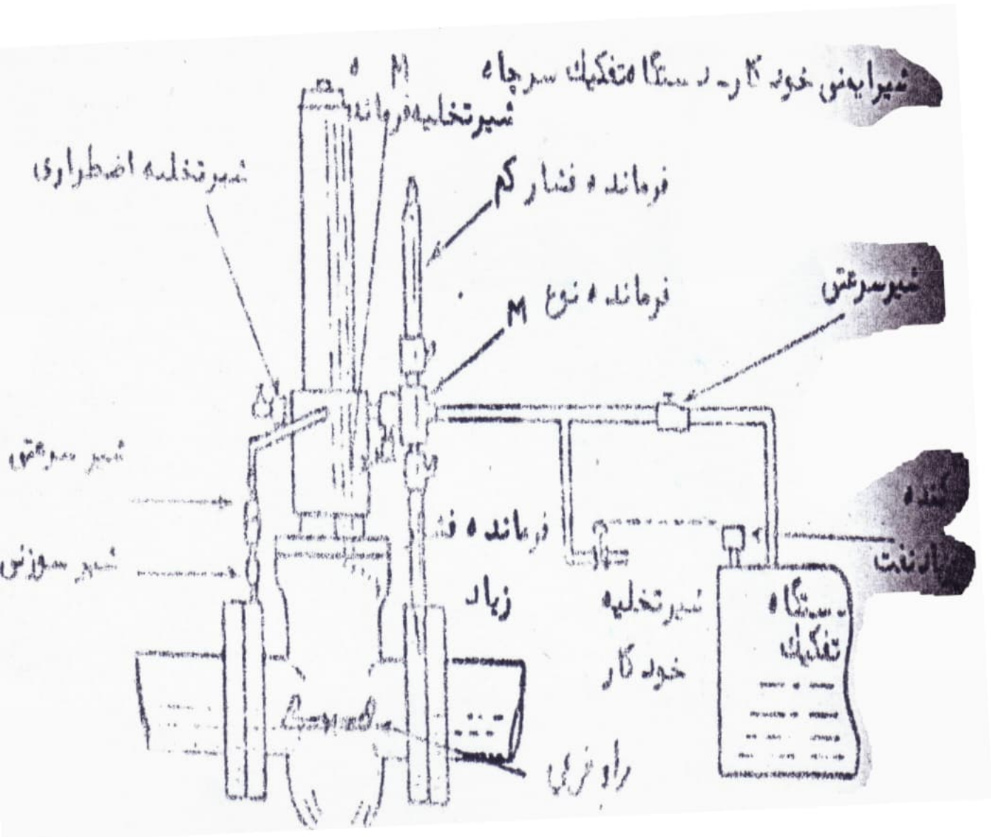
شکل ۳ ساختمان شیر ایمنی خودکار
